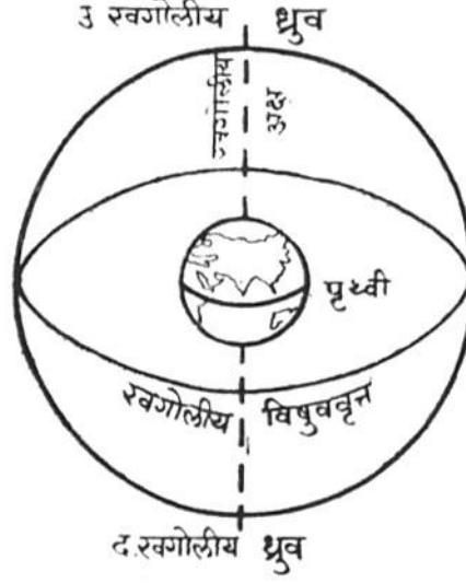
आकृती क्र. १२ : खगोल
