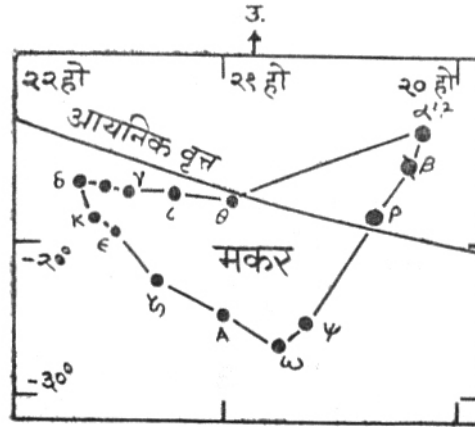
आकृती क्र. ३५ : मकर राशी
