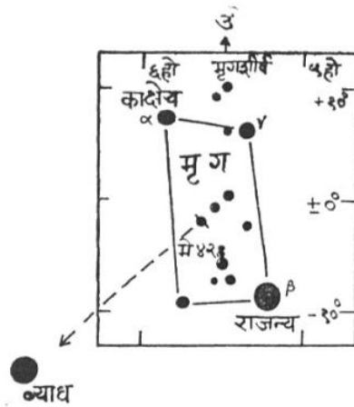
आकृती क्र. २४ : मृग व मृगशीर्ष
