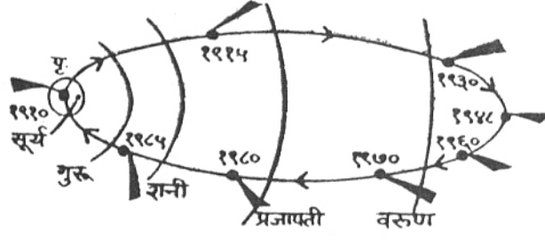
आकृती क्र. ६२ : हॅलेचा धूमकेतू
