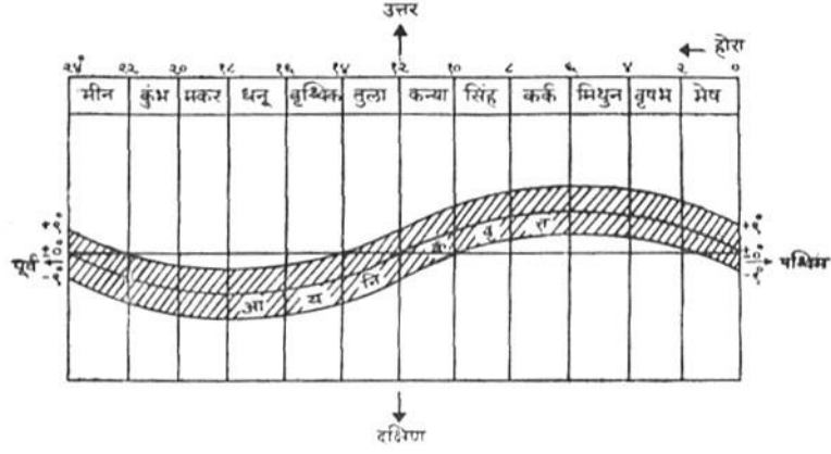
आकृती क्र. १८ : ग्रहमार्ग
