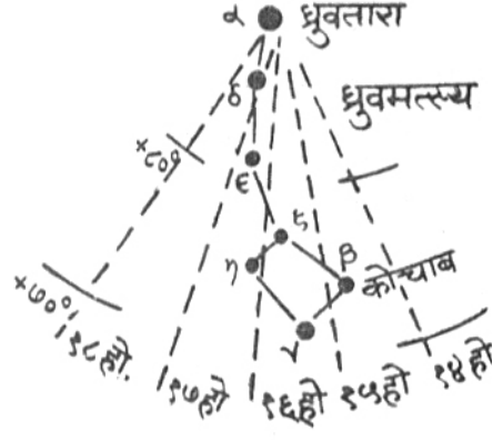
आकृती क्र. ४३ : ध्रुवमत्स्य
